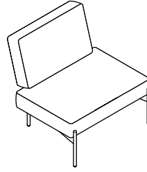
TI1PN L: 850 P: 780 HT: 810 HS: 420
